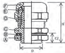
外形寸法一覧表(メタルケーブルグランド)
